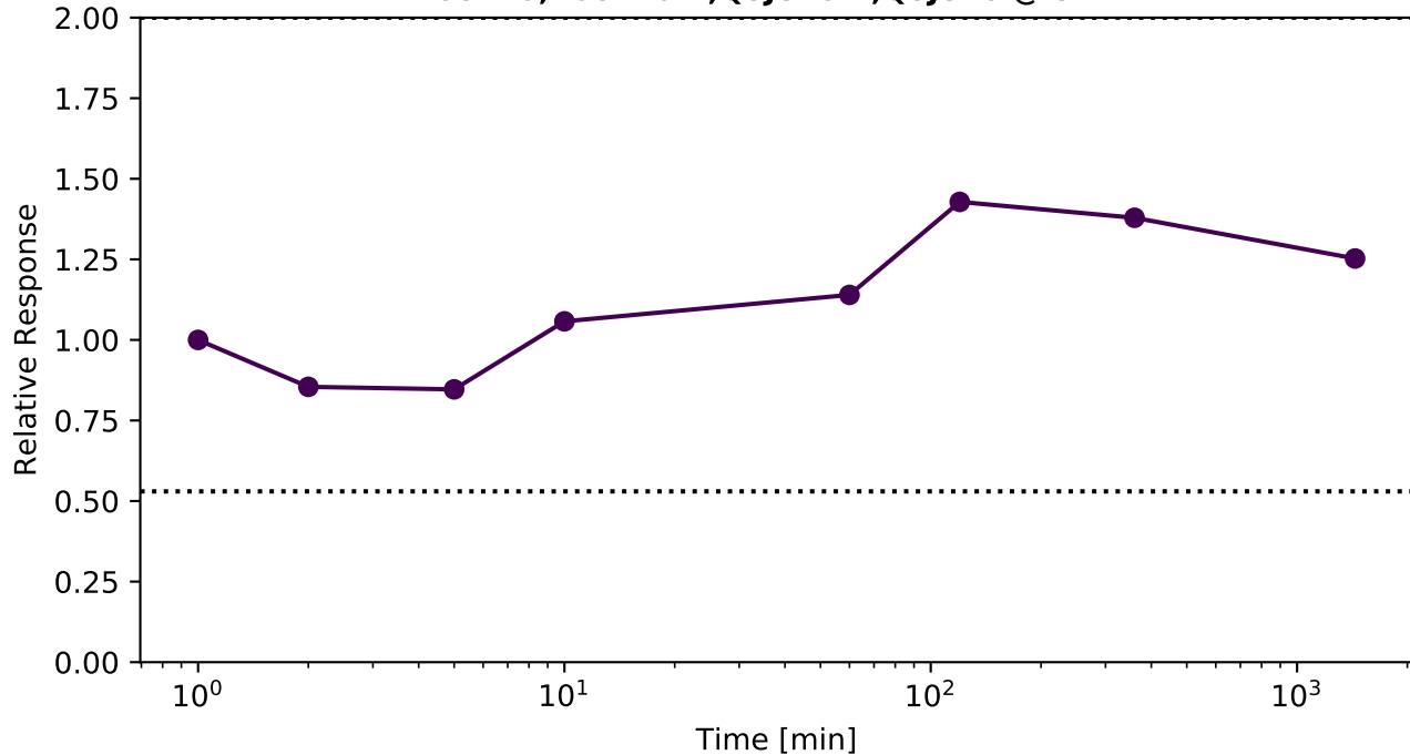
P08240;P08240-2;Q5JST6-2;Q5JST6 @ SRPR
