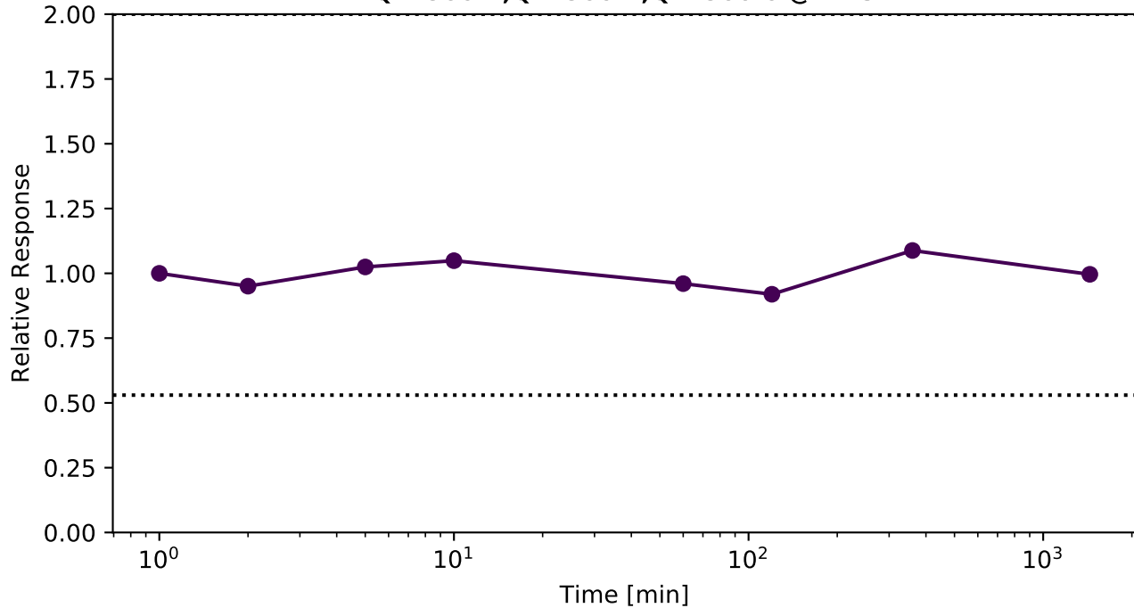
Q12906-7;Q12906-4;Q12906-6 @ ILF3
