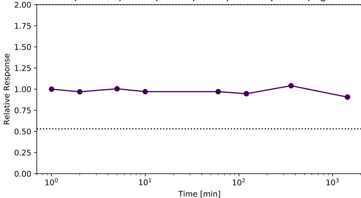
P29218;P29218-3;H0YBL1;E5RG13;E5RIP7;P29218-2;E5RG94;.. @ IMPA1
