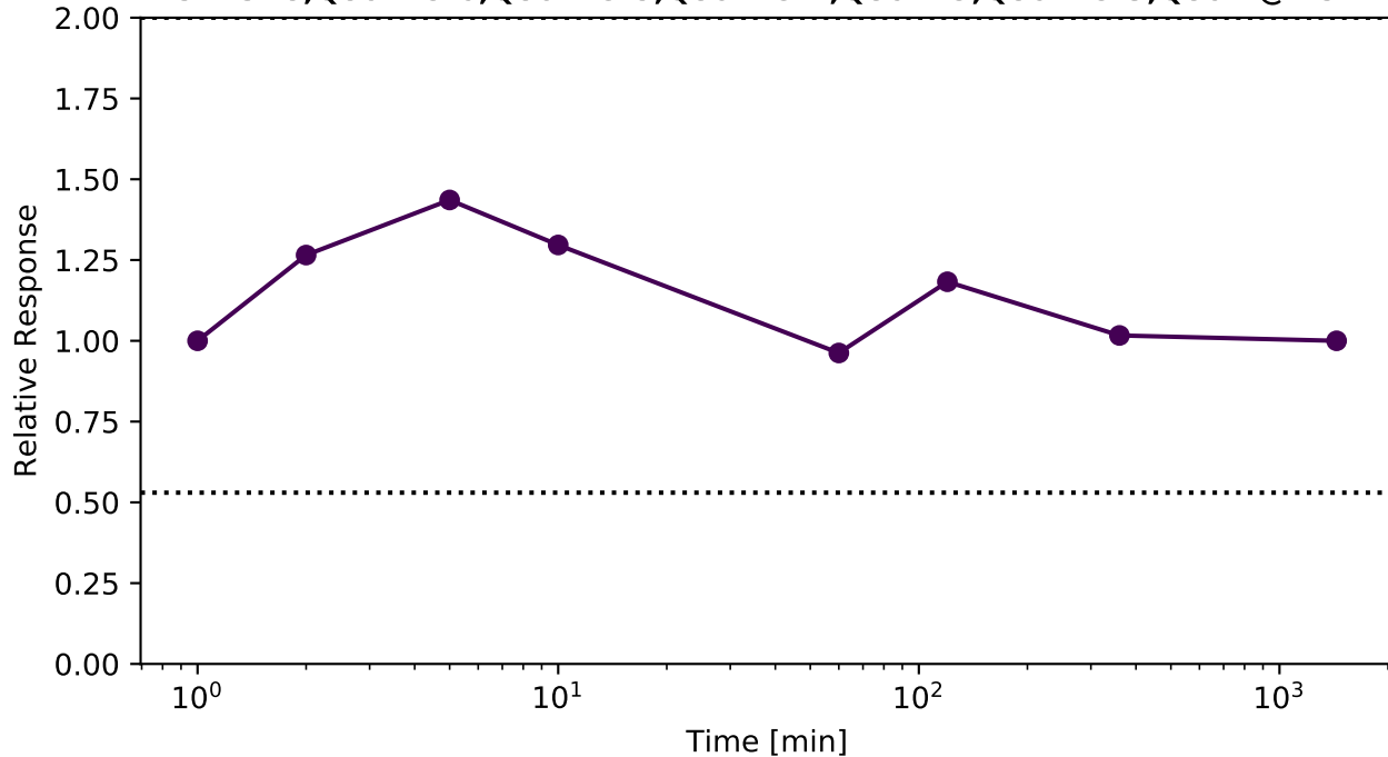
S4R3V8;Q86X29-6;Q86X29-5;Q86X29-4;Q86X29;Q86X29-3;Q86.. @ LSR
