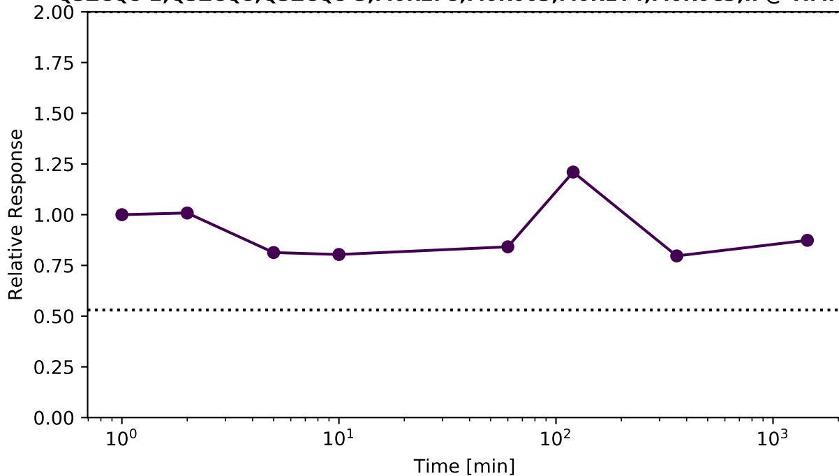
Q3ZCQ8-2;Q3ZCQ8;Q3ZCQ8-3;M0R2F8;M0R003;M0R1Y4;M0R0C3;.. @ TIMM50
