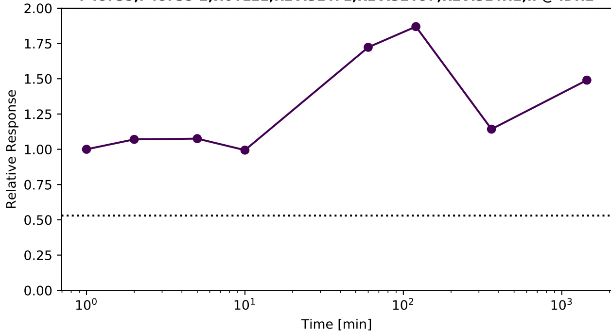
P48735;P48735-2;H0YL11;REVI3L471;REVI3L4U7;REVI3L4H1;.. @ IDH2
