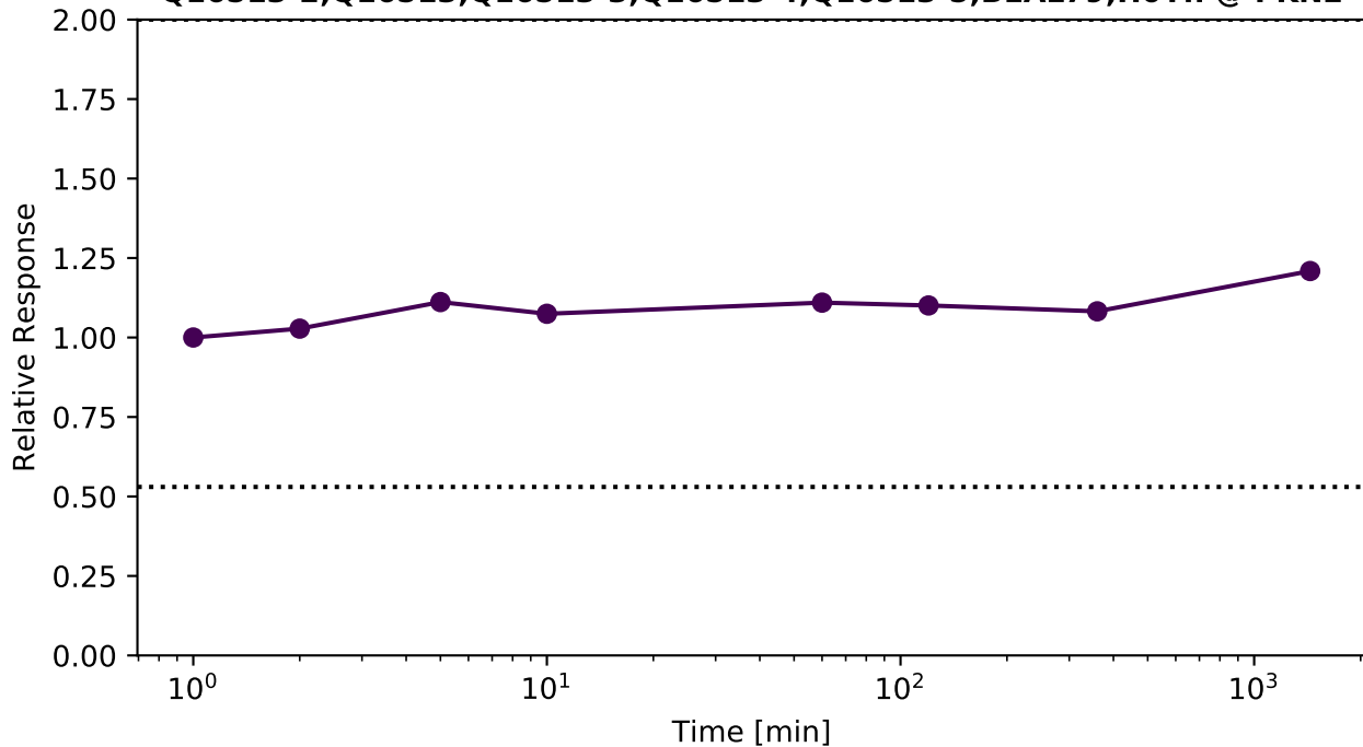
Q16513-2;Q16513;Q16513-3;Q16513-4;Q16513-5;B1AL79;H0Y.. @ PKN2
