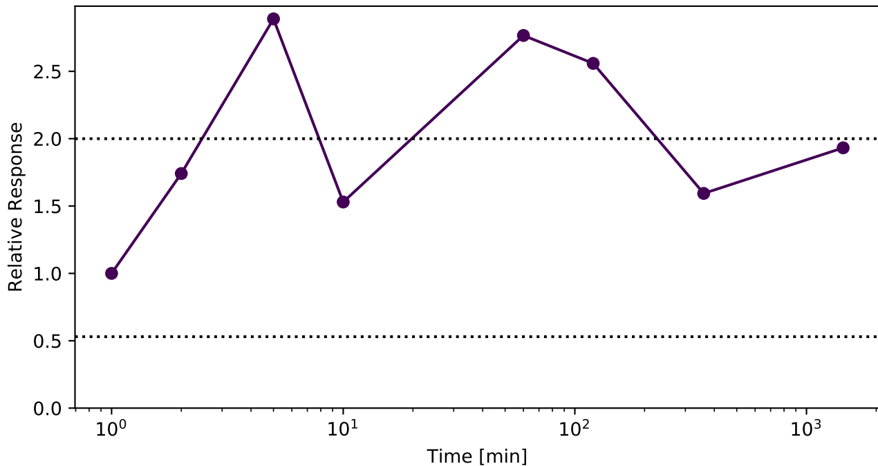
A0A1W2PRX1 @ nan
