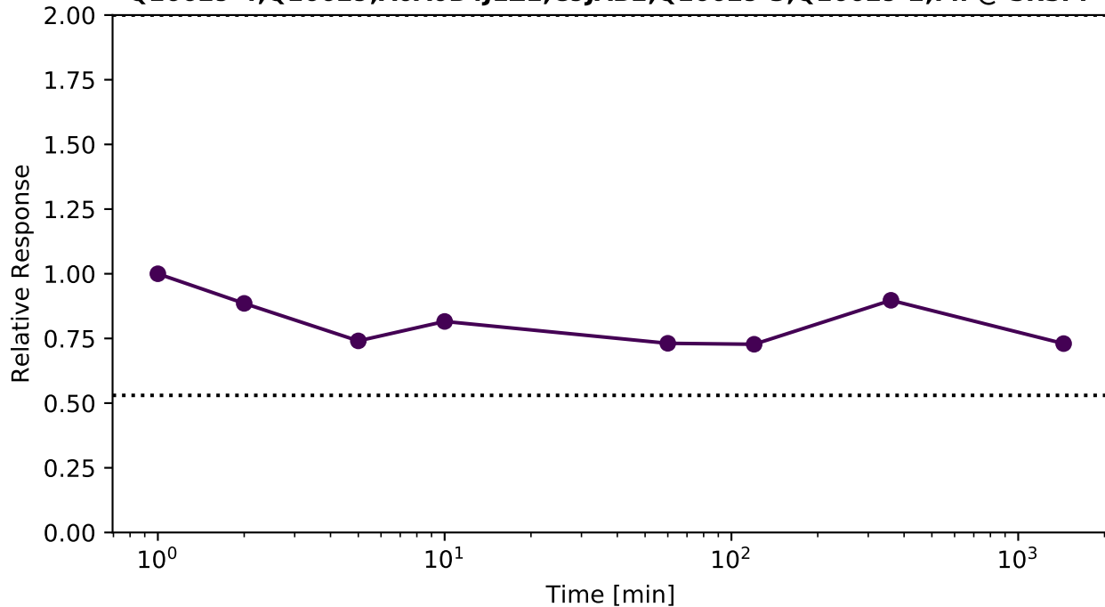
Q16629-4;Q16629;A0A0B4J1Z1;C9JAB2;Q16629-3;Q16629-2;F.. @ SRSF7
