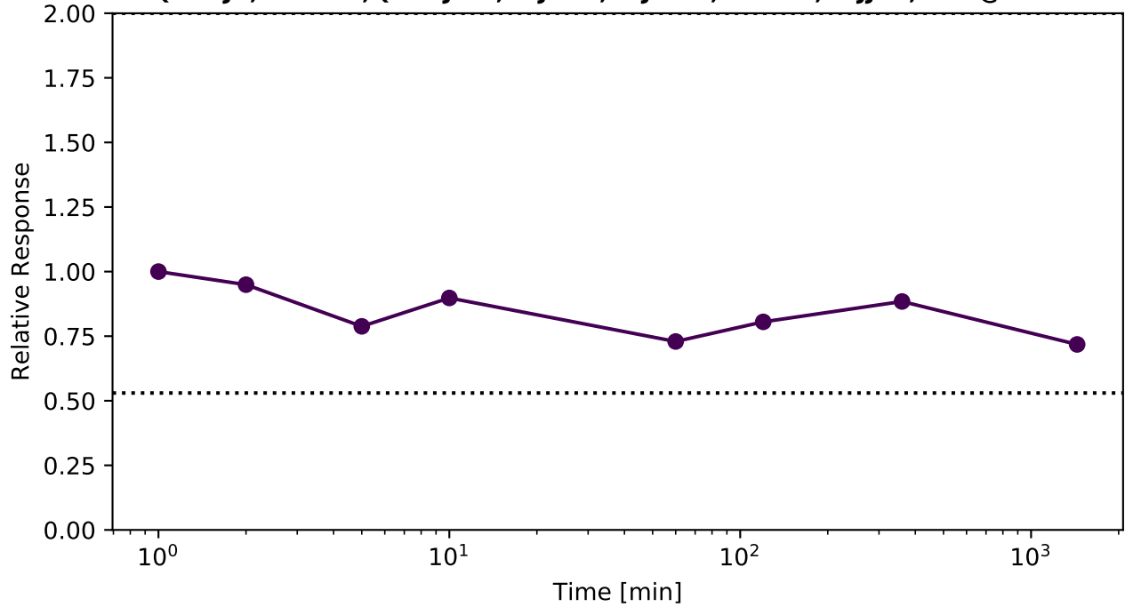
Q9NTJ3;E9PD53;Q9NTJ3-2;C9JR83;C9JWF0;C9IYK2;C9JJ64;C9.. @ SMC4
