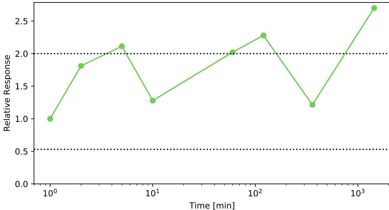
R4GND0;Q9NQ25-4;Q9NQ25-6;Q9NQ25-5;Q9NQ25-3;Q9NQ25 @ SLAMF7
