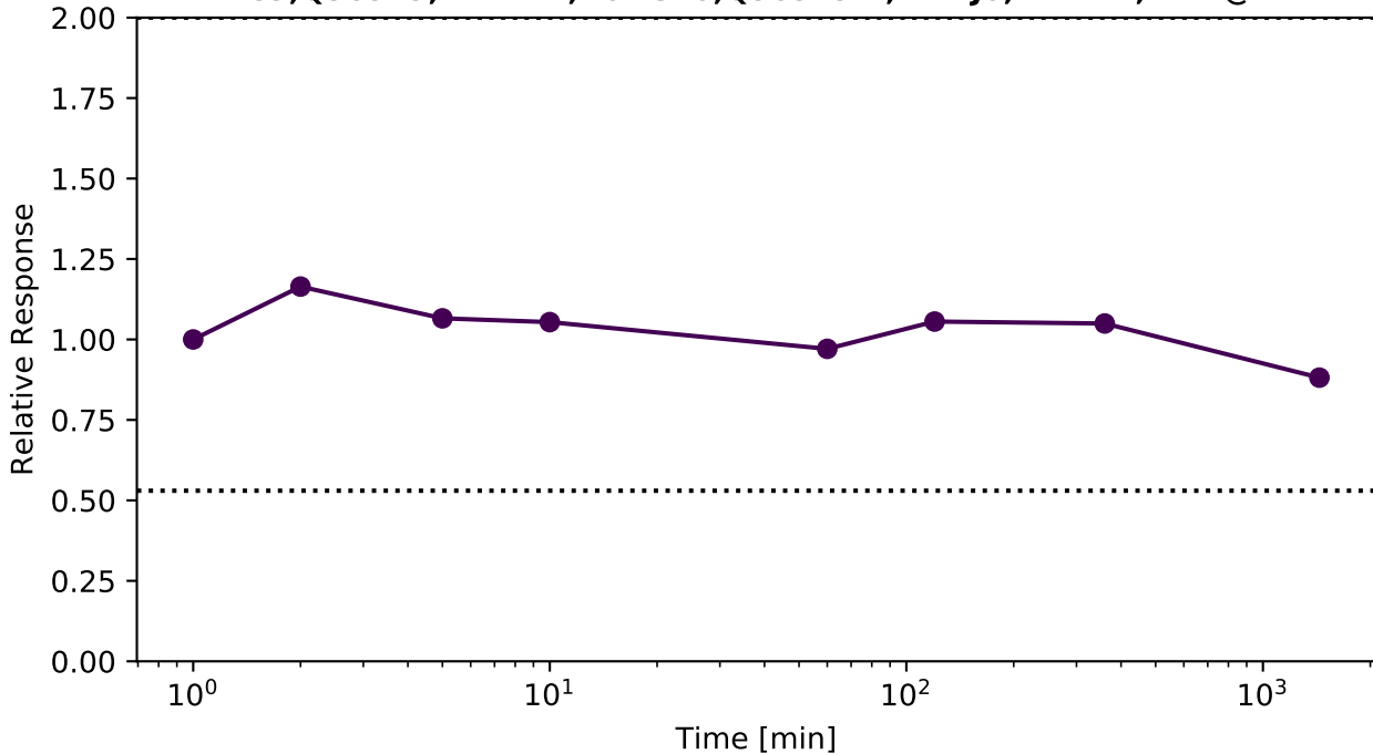
K7EMC9;Q969T9;K7ENL2;A6NG10;Q969T9-2;K7EIJ0;K7EIN1;K7.. @ WBP2
