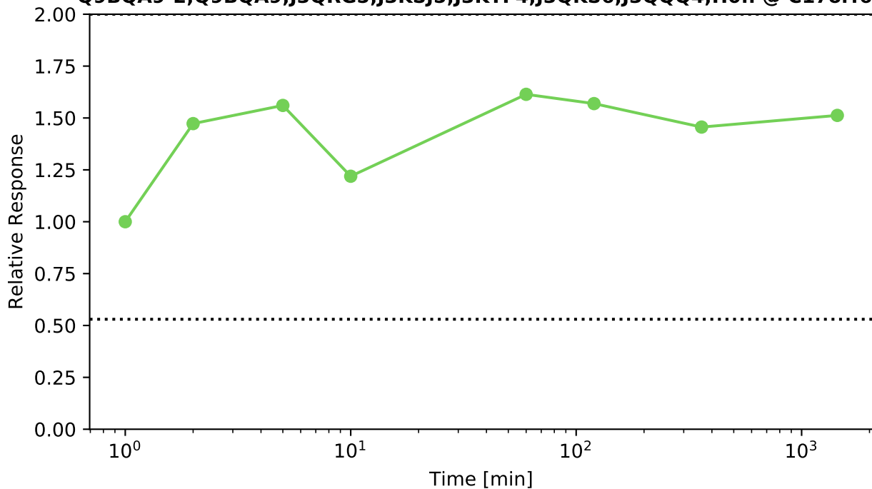
Q9BQA9-2;Q9BQA9;J3QRG5;J3KSJ5;J3KTF4;J3QKS6;J3QQQ4;H0.. @ C17orf62
