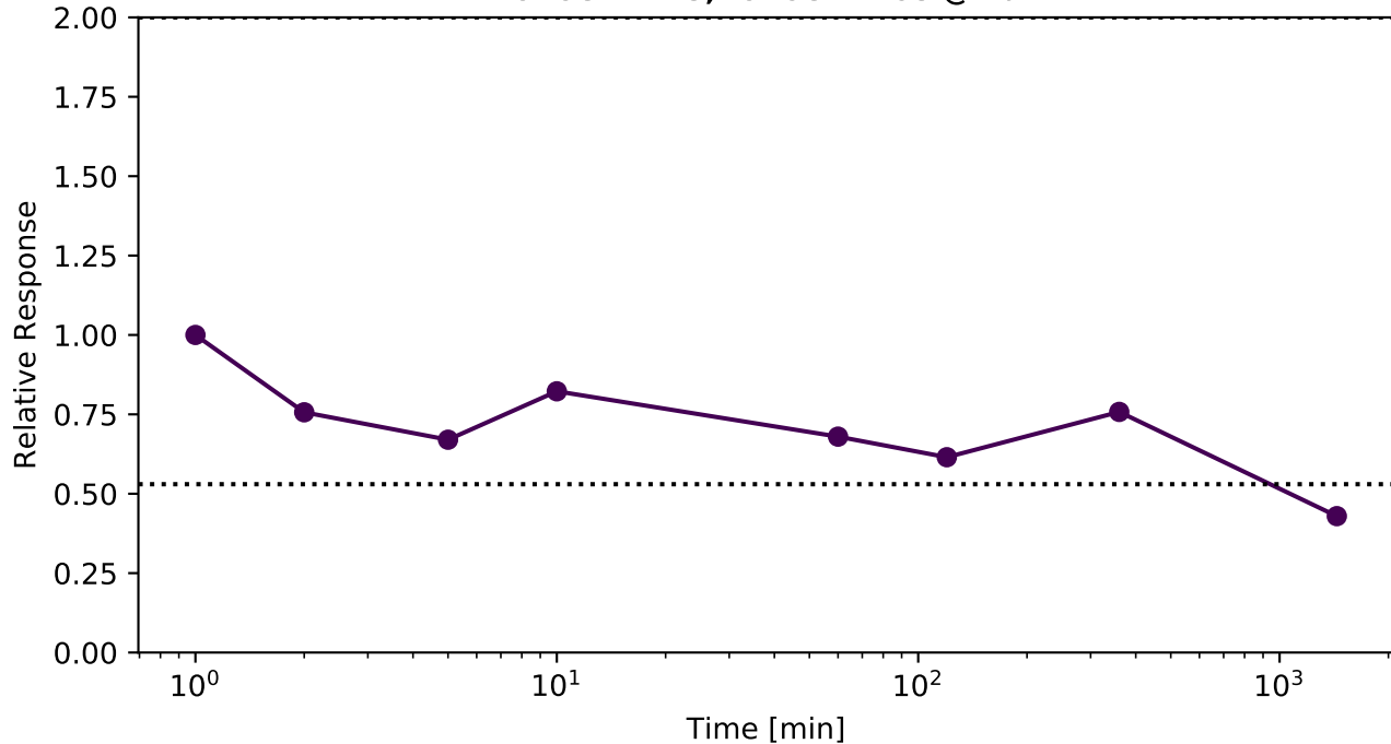
A0A0U1RRE5;A0A0U1RR68 @ nan
