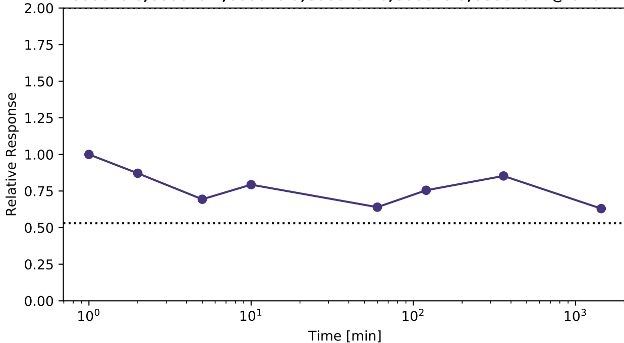
O95628-8;O95628-4;O95628-9;O95628-10;O95628-3;O95628-.. @ CNOT4
