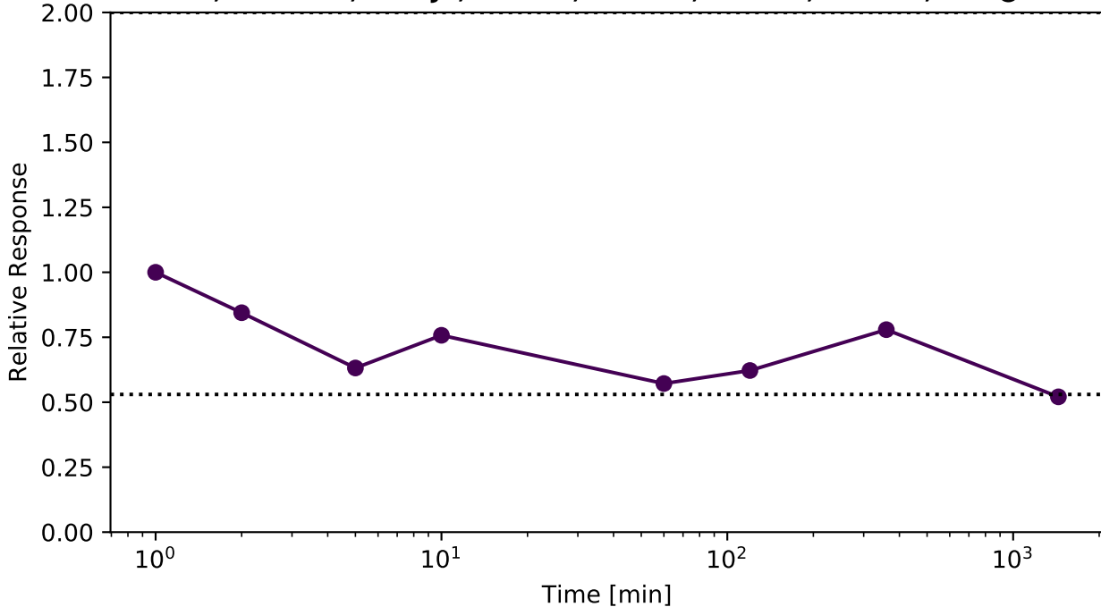
P32321;P32321-2;D6RBJ9;D6R9S0;D6RBN2;D6RC36;D6RAR9;D6.. @ DCTD
