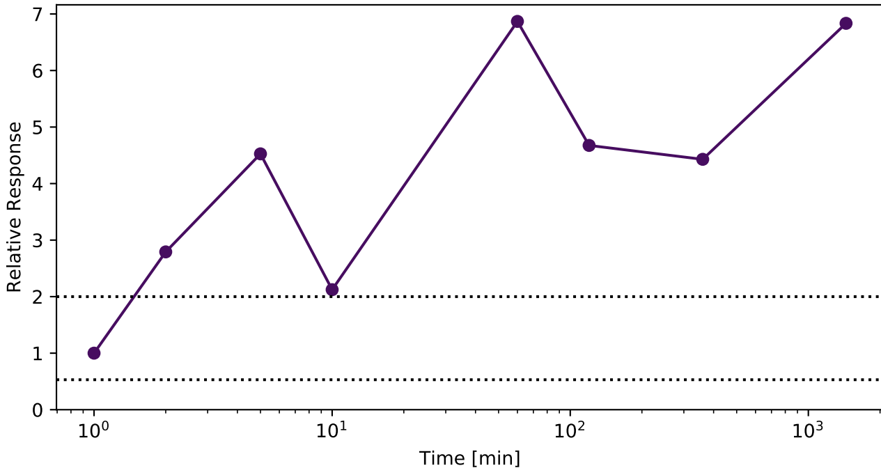
F8VU90;Q9NYL4-2;Q9NYL4;H0YHM7 @ FKBP11
