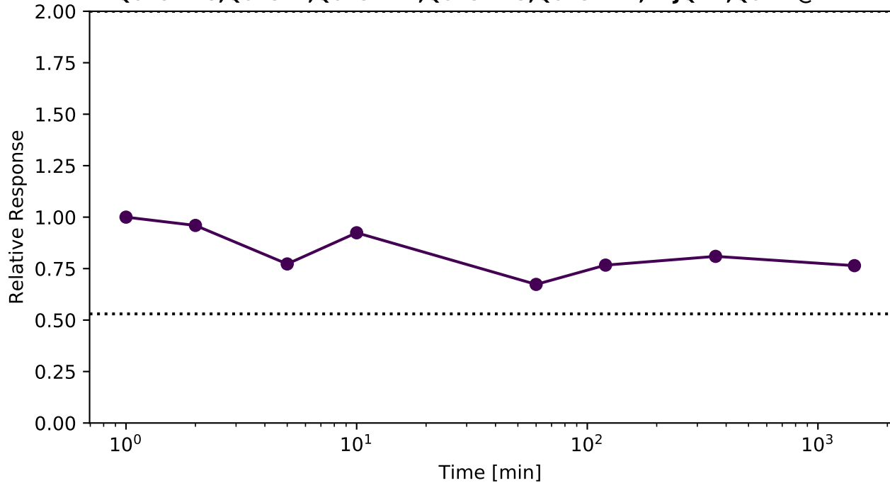
Q07812-8;Q07812;Q07812-2;Q07812-5;Q07812-7;K4JQN1;Q07.. @ BAX
