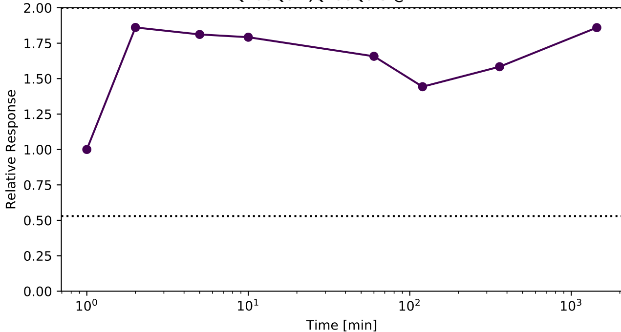
Q70UQ0-4;Q70UQ0-3 @ IKBIP
