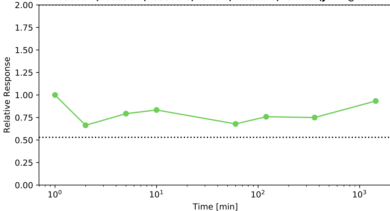
P53990-2;P53990-4;P53990-5;H3BUI0;P53990-3;H3BMU1;J3K.. @ IST1
